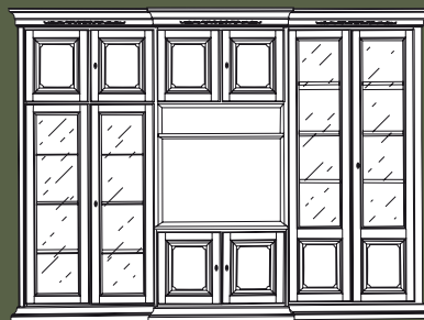
Art. 0731/A Composizione intagliata L. 328 P. 58 H. 242 Pag. 43 Peso kg 180,00 - mc 2,82
