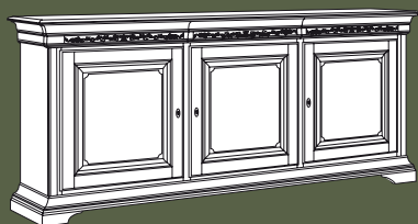
Art. 0710 Credenza 3 porte intagliata L. 228 P. 52 H. 100 Pag. 14-15 Peso kg 95,00 - mc 1,3
