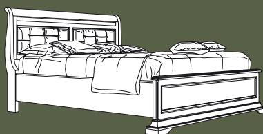
Art. 0780 Letto liscio con contenitore, rete a doghe e pannelli da tappezzare L. 180 P. 208 H. 114 Peso kg 110,00 - mc 0,9
