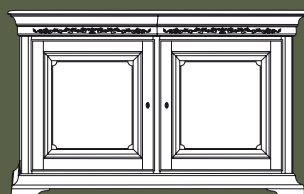
Art. 0707 Credenza 2 porte intagliata L. 158 P. 52 H. 100 Pag. 13 Peso kg 55,00 - mc 0,9
