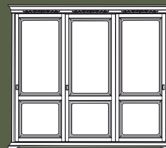
Art. 0726 Armadio 3 ante scorrevoli intagliato L. 284 P. 64 H. 247 Pag. 50 Peso kg 130,00 - mc 1,1
