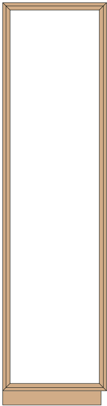
Art. C4/P Colonna singola DX cm. L. 57 - P. 37 - H. 225
