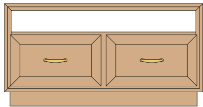
Art. C6/P Base 2 cestoni 1 vano a giorno cm. L. 110 - P. 52 - H. 62
