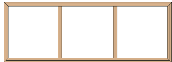
Art. C8/P Pensile 3 ante cm. L. 163 - P. 37 - H. 57
