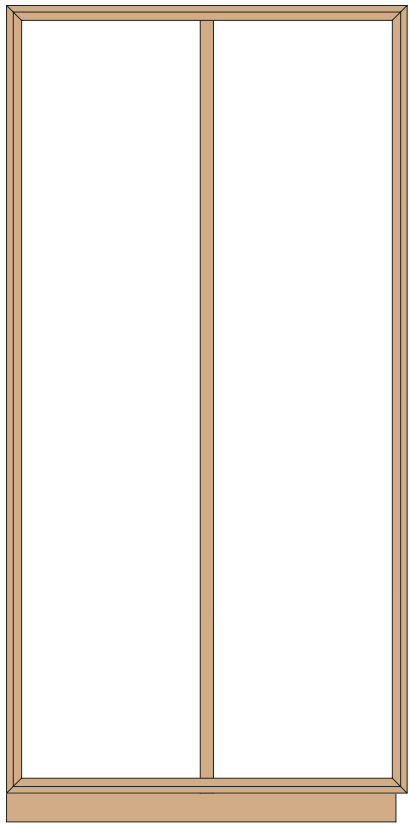
Art. C2/P Colonna doppia DX cm. L. 110 - P. 37 - H. 225
