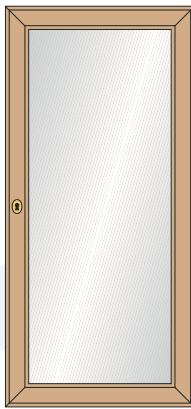
Art. C19/P Porta lunga con vetro cm. L. 52 - H. 105
