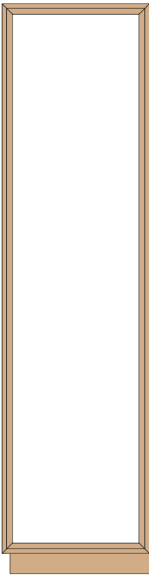
Art. C3/P Colonna singola SX cm. L. 57 - P. 37 - H. 225
