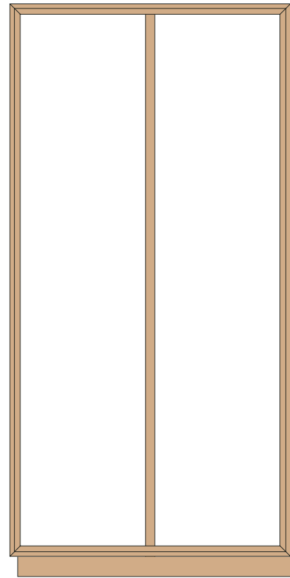
Art. C1/P Colonna doppia SX cm. L. 110 - P. 37 - H. 225
